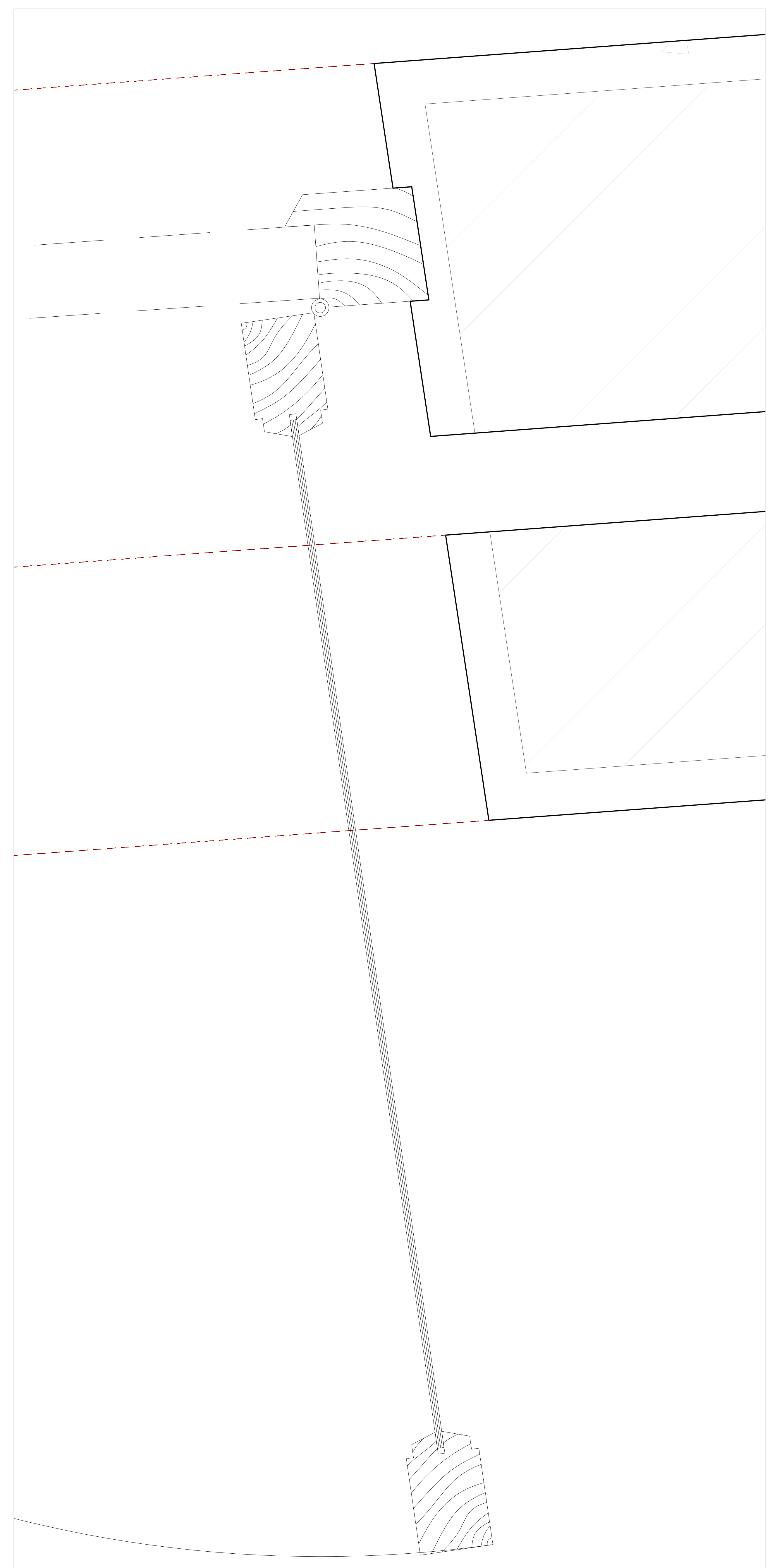
Pormenor do caixilho da janela 1:1
