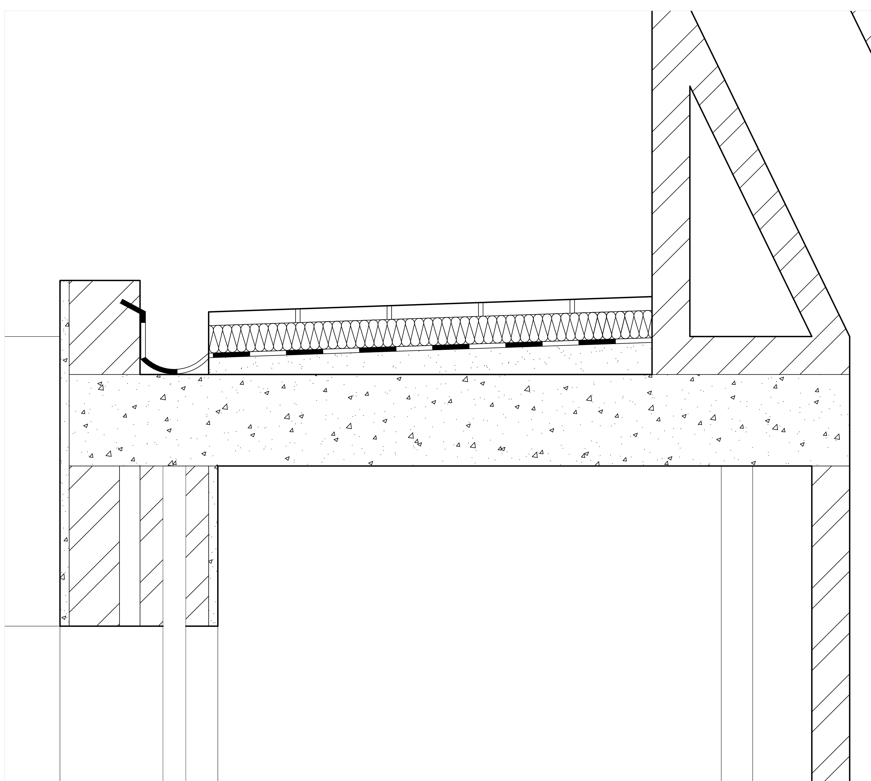
Pormenor cobertura 1:5
