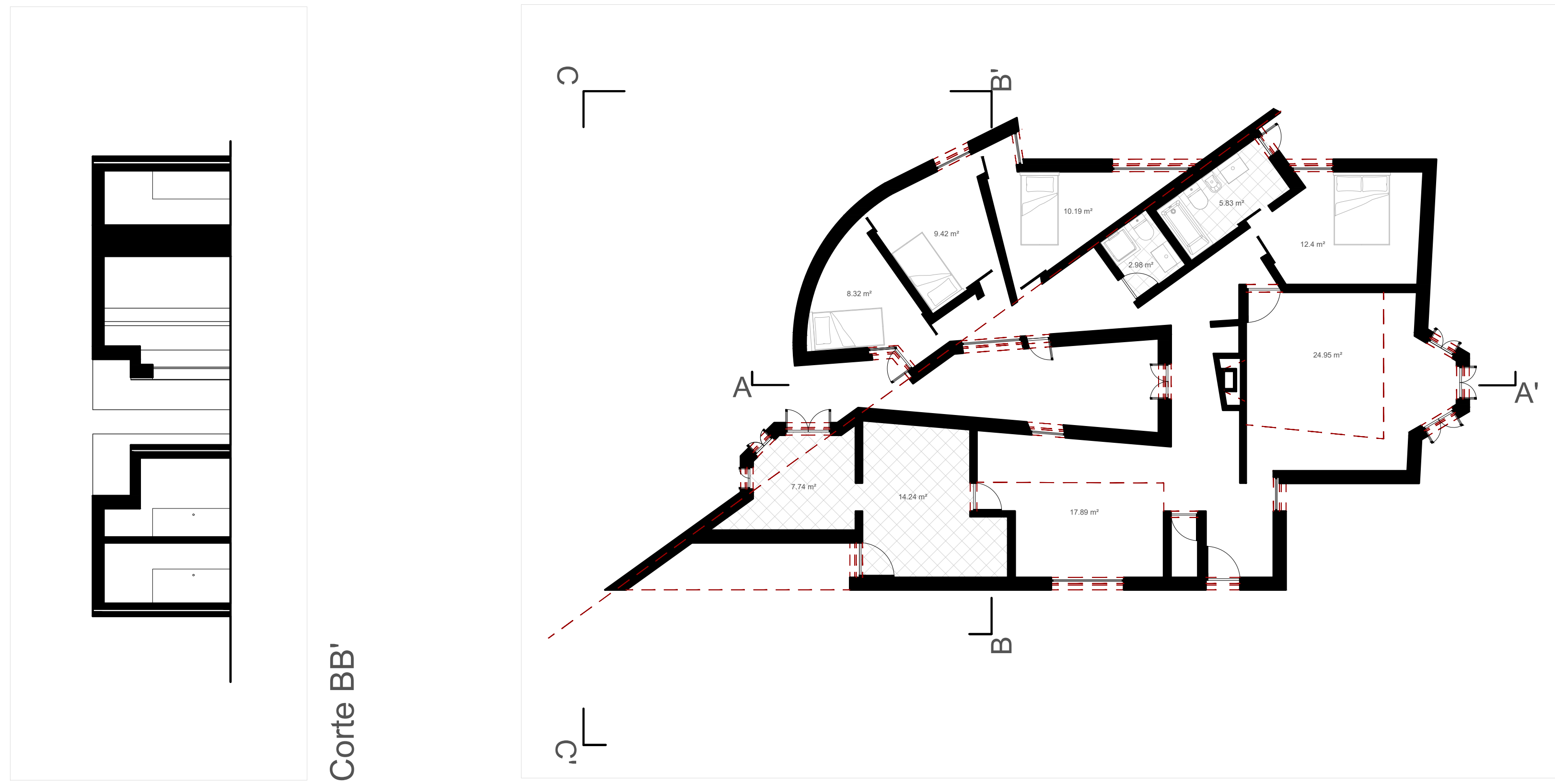
Planta geral 1:100
